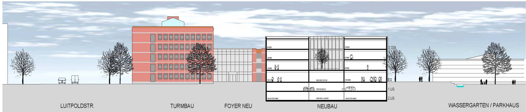
LÄNGSSCHNITT
